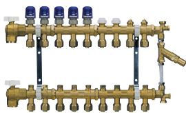
Vario B (WGF) -jakotukki (runko 1") 1999 alkaen
