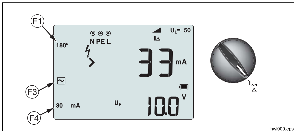
Taulukko 17. Vikavirtasuojan laukaisuvirta / Kytkin- ja liitinasetukset
