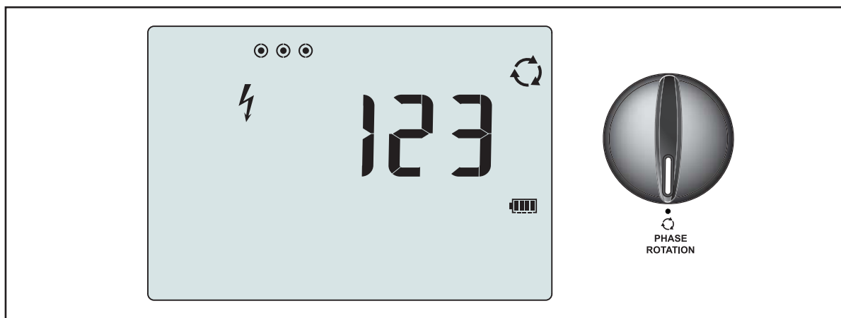
Kuva 11. Vaihejärjestysnäyttö
