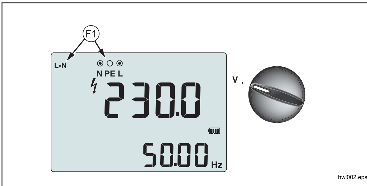
Taulukko 11. Jännitenäyttö/Kytkin- ja liitinasetukset
