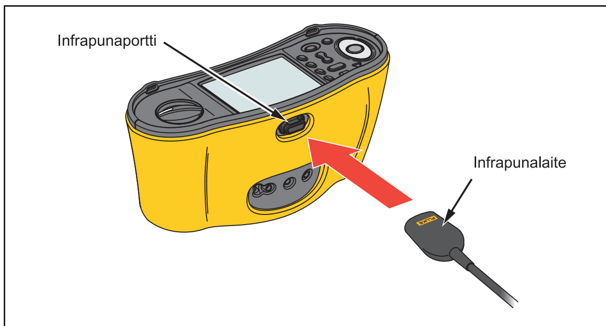
Kuva 16. IR-sarjakaapelin liitântä
