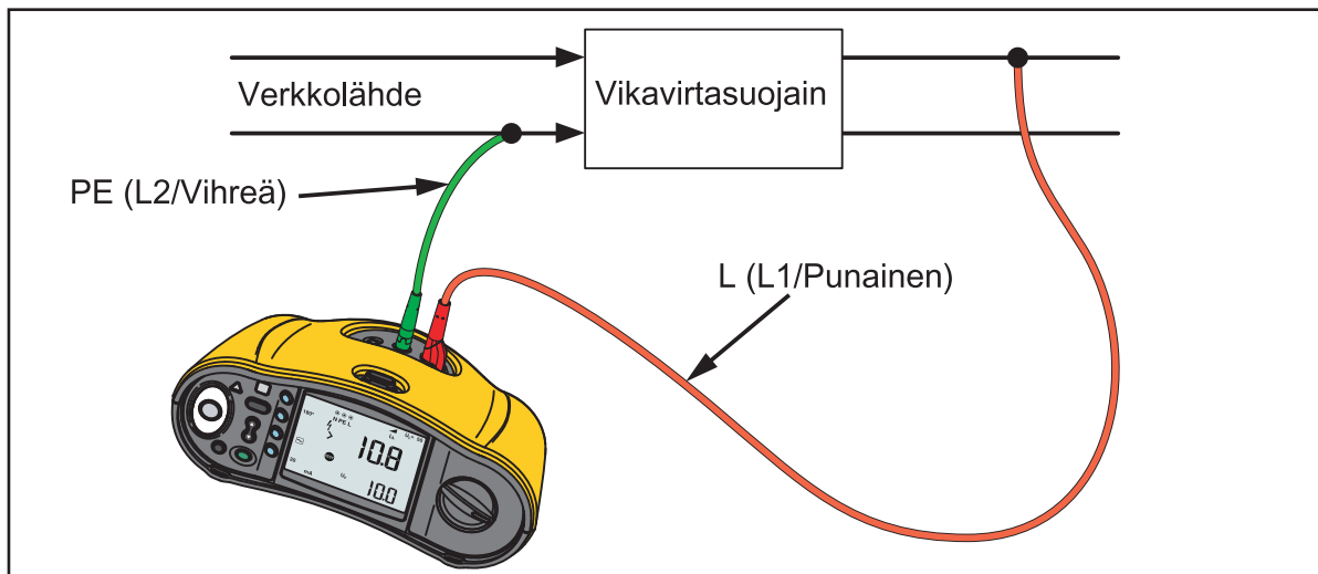
Taulukko 8. Kytkenä vikavirtasuojan testauksessa IT:n sähköisissä järjestelmissä
