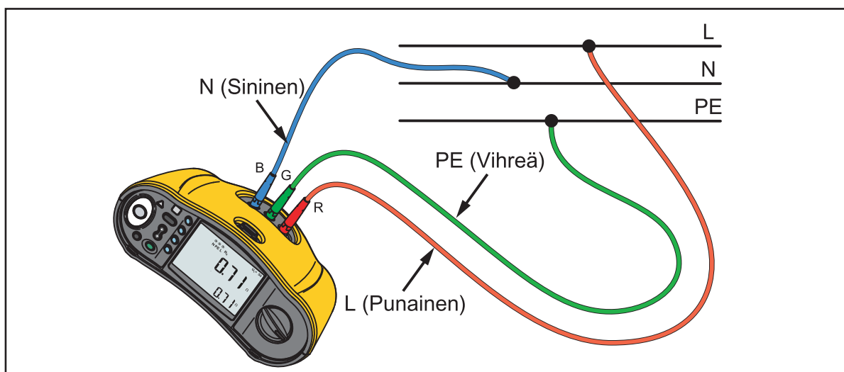
Kuva 13. 3-johtoinen kytkentä maadoitusresistanssin silmukkatestiä varten (ei laukaisutilaa)
