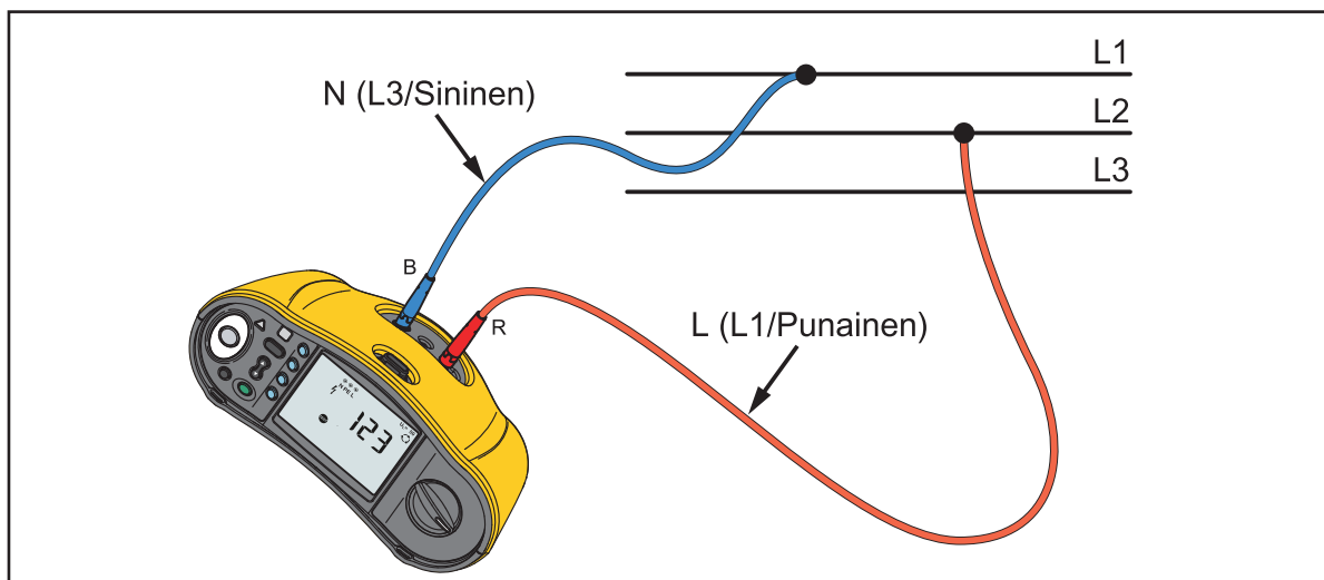
Kuva 7. 3-vaihejärjestelmän mittaus
