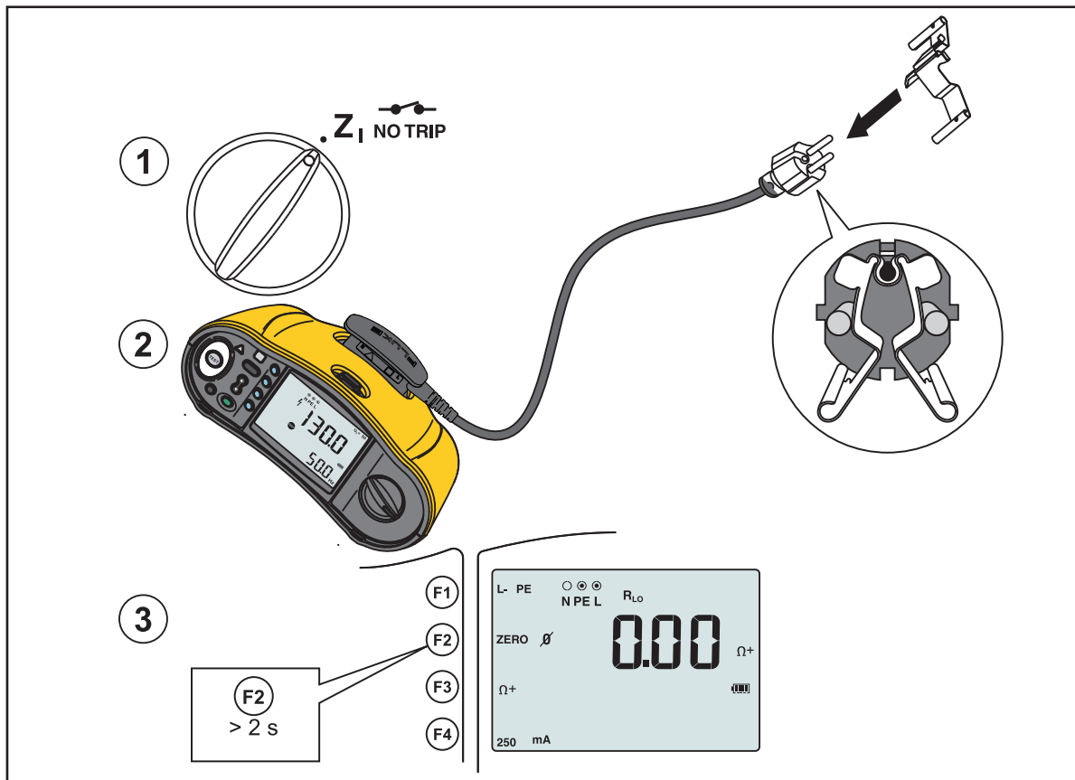
Kuva 2. Nollausnäyttö
