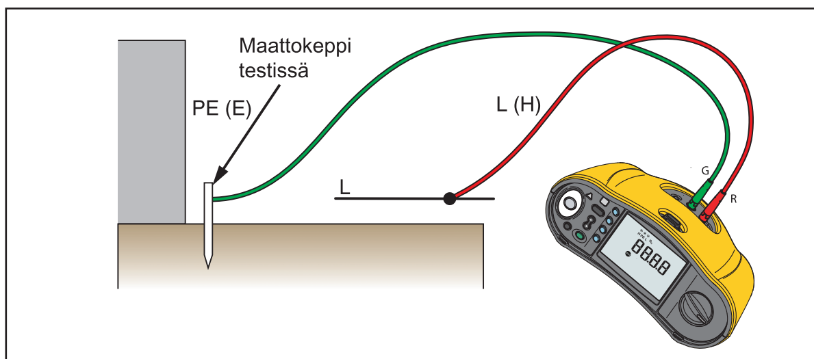
Kuva 14. 2-johtoinen kytkentä maadoitusresistanssin silmukkatestiä varten (suuren virran laukaisutila)
