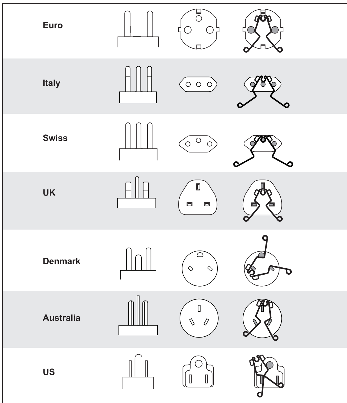
Kuva 3. Maakohtaiset nollausadapteriasetukset
