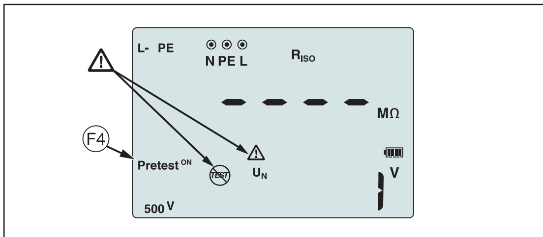
Kuva 5. Turvallisuuden esitesti näyttö
