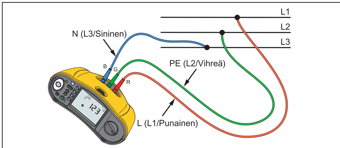
Kuva 10. Vaihejärjestystestin kytkentä
