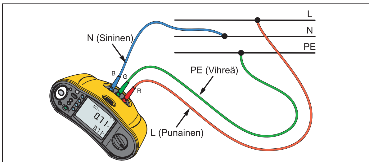
Kuva 4. Turvallisuuden esitestin liitännät
