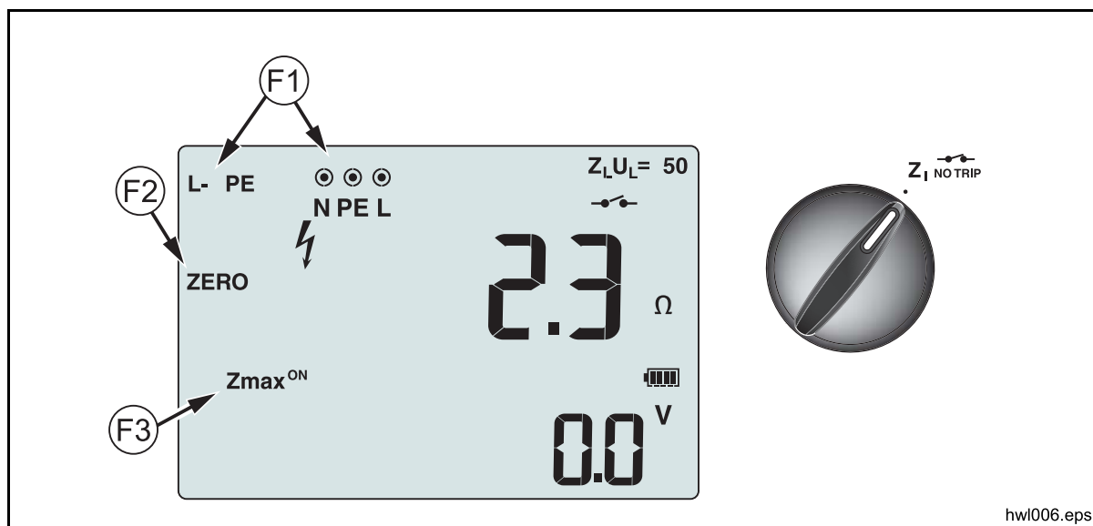
Taulukko 14. Silmukka-/linjaimpedanssi/Kytkin- ja liitinasetukset
