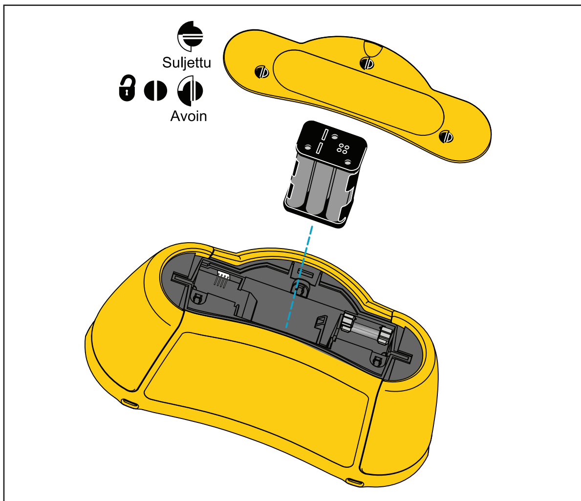
Kuva 17. Pariston vaihto
