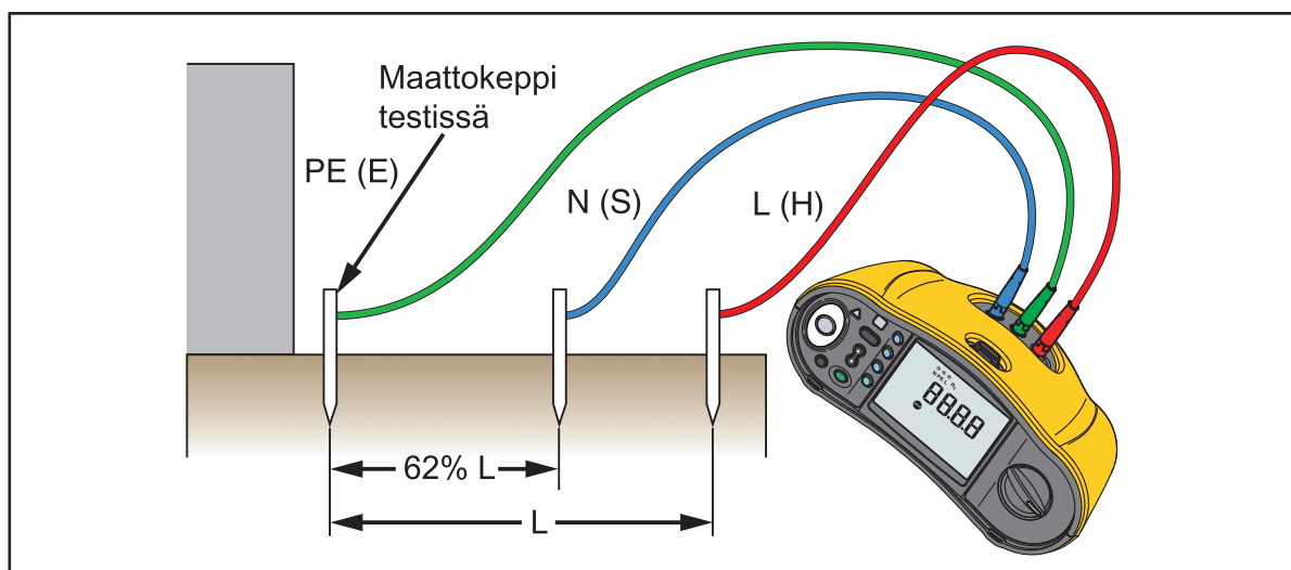
Kuva 12. Maadoitusresistanssitestin kytkentä
