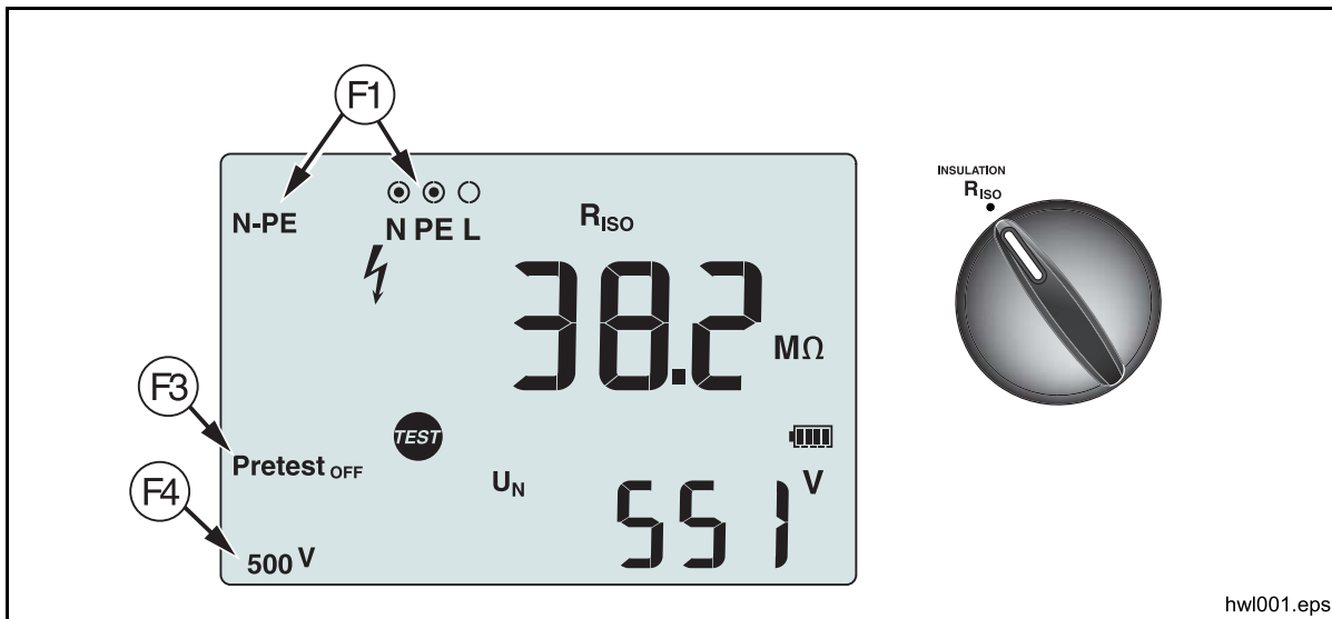
Taulukko 12. Eristysvastuksen näyttö / Kytkin- ja liitinasetukset
