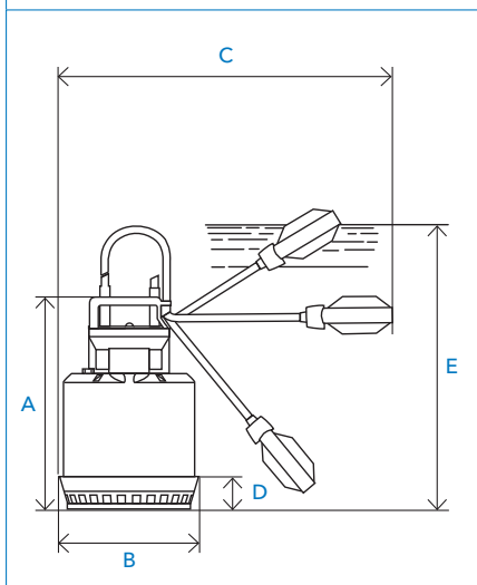
Mittakuva: SX 2-3
