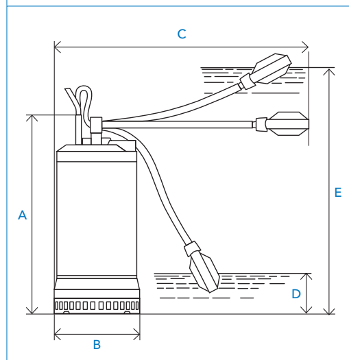
Mittakuva: SX 5-15
