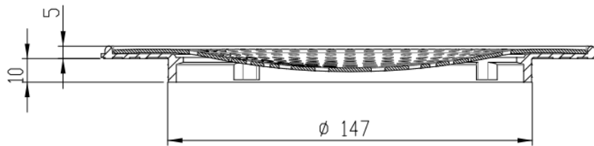
SECTION A-A SCALE 1 : 2
