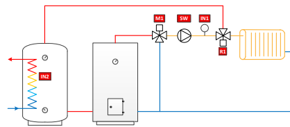
7. 1-circuit and DHW VO
