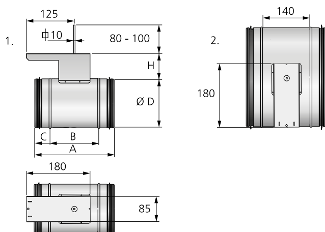
Kuva 2. CRT, mitat.
