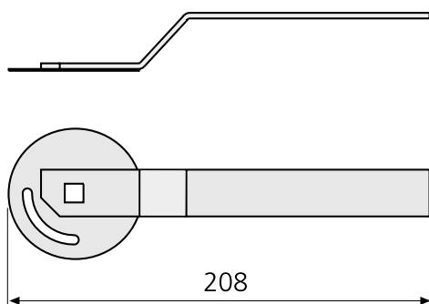
Kuva 3. Säätkahva CRTT-1.
