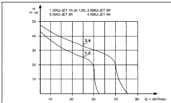
ISKU-Jet pumput, tehokäyrästä
