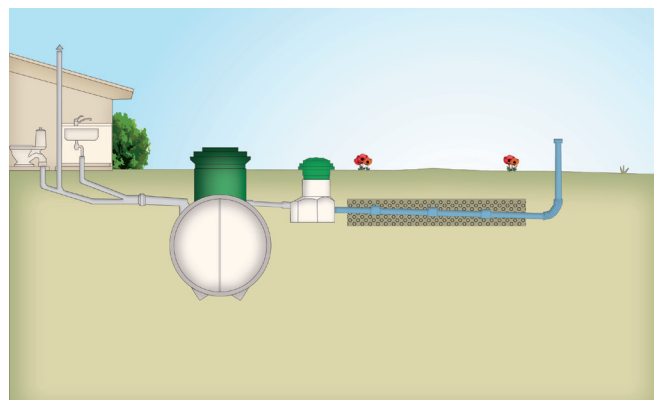
Imeytysputkistopaketti LVI-nro: 3625 430
