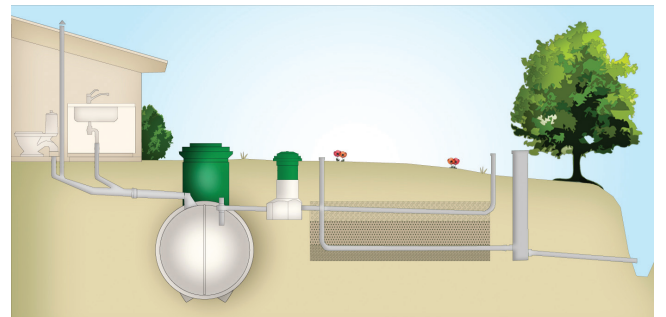
Suodatusputkistopaketti LVI-nro: 3625 430 + 3625 520
