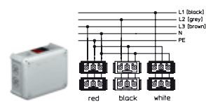
Kolmenapainen Wieland, kolmivaiheinen T 100 WB 6S 3x2 OBO 2007 81 4 Wieland 3x2 (va; mu; pun)
