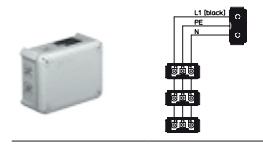
Wieland-liittimelliset T100 WS 1S3 3S3A OBO 2007 87 0
