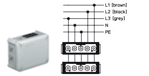
Viisinapainen Wieland, kolmivaiheinen T 100 WB 2s5 OBO 2007 85 2
