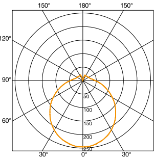
Valonjakokäyrä RS PRO LED B1 varavalo
