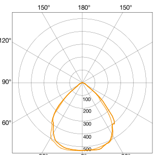
Valonjakokäyrä RS PRO DL LED 14 W
