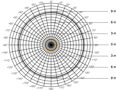
Toiminta-alue L 676 LED Asennuskorkeus 2,8 m Musta = tangentiaalinen kulkusuunta Oranssi = säteittäinen kulkusuunta
