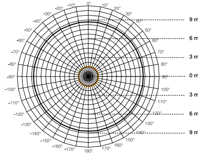
Toiminta-alue L 321 wave Asennuskorkeus 2,8 m Musta = tangentiaalinen kulkuasuunta Oranssi = säteittäinen kulkuasuunta
