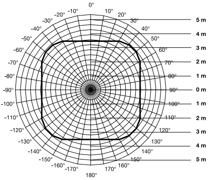
Tunnistusalue IR Quattro Slim Asennuskorkeus 2,80 m Musta = tangentiaalinen, radiaalinen ja läsnäolo
