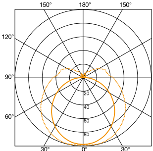
— C0 / C180 cd/1000lm — C90 / C270 Valonjakokäyrä BRS 85P · 86L · 87L
