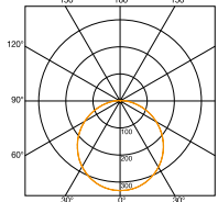
Valonjakokäyrä RS PRO LED S1 PC
