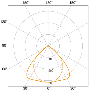
Valonjakokäyrä RS PRO 4100
