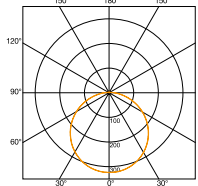
Valonjakokäyrä RS PRO LED S1 lasi
