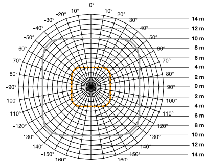
Tunnistusalue IR Quattro HD Asennuskorkeus 2,80 m Harmaa = tangentiaalinen Oranssi = säteittäinen Musta = läsnäolo
