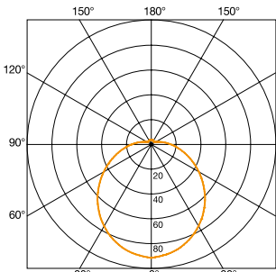
Valonjakokäyrä RS PRO 1000 2x18W
