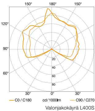
Valonjakokäyrä L 400S
