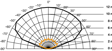
Toiminta-alue IS2160 ECO Asennuskorkeus 1,8 m Musta = tangentiaalinen kulkusuunta Oranssi = säteittäinen kulkusuunta
