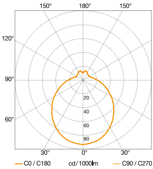
Valonjakokäyrä RS PRO 500
