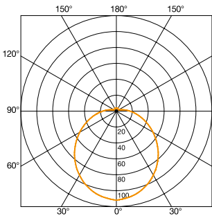
Valonjakokäyrä RS PRO 2000 2 x 26W
