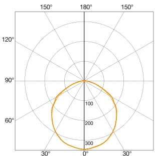
Valonjakokäyrä RS PRO LED S1 IP65 C0 / C180 cd / 1000lm C90 / C270
