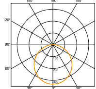
Valonjakokäyrä RS PRO LED S1 PMMA
