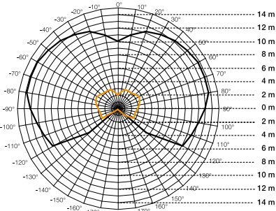
Toiminta-alue L 400S · L 410S Asennuskorkeus 2,8 m Musta = tangentiaalinen kulkusuunta Oranssi = säteittäinen kulkusuunta
