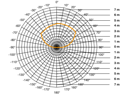
Toiminta-alue BRS 85P · 86L · 87L Asennuskorkeus 2,8 m Oranssi = säteittäinen kulkusuunta
