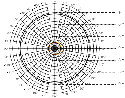
Toiminta-alue L 691 LED Asennuskorkeus 2,8 m Musta = tangentialinen kulkusuunta Oranssi = säteittäinen kulkusuunta
