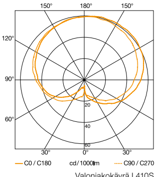
Valonjakokäyrä L 410S
