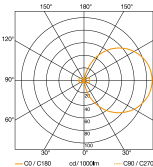
Valonjakokäyrä L 321 wave
