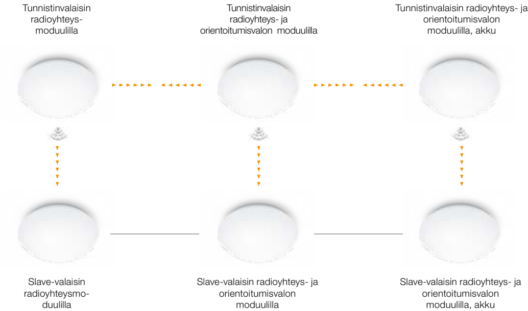
Langattoman tiedonsiirron suunta tunnistimesta tunnistimeen tai slave-valaisimeen Yhdistämismahdollisuus johdottamalla (enint. 5 x RS PRO 500)
