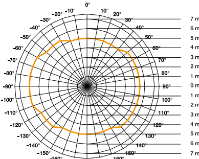
Toiminta-alue RS PRO LED S1 IP65 Asennuskorkeus 2,8 m Oranssi = säteittäinen kulkusuunta
