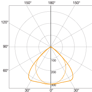
Valonjakokäyrä RS PRO 4000
