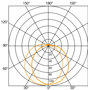
Valonjakokäyrä RS PRO 2000 1 x 26W
