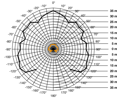
Toiminta-alue sensIQ Asennuskorkeus 1,8 m Musta = tangentiaalinen kulkusuunta Oranssi = säteittäinen kulkusuunta
