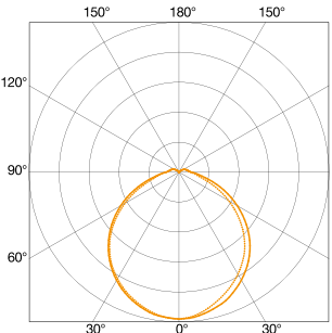
Valonjakokäyrä L691LED C0 / C180 cd / 1000lm C90 / C270
