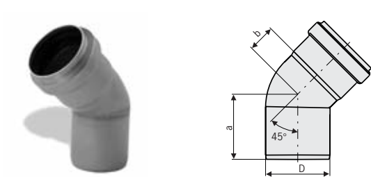
45° kulmayhteet
