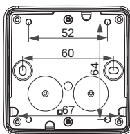
AP9 pohjaosa
