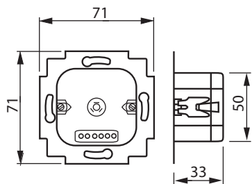
Releyksiköt
